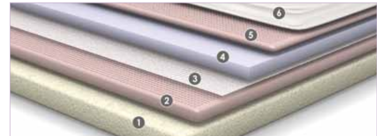
1. Bloque HR (13 cm) 2. Viscoelástica D-80 (7 cm) 3. Textil NT 4. Sistema Commodo+® 5. Viscoelástica 6. Tapicería Stretch con tecnología Optigrade®
