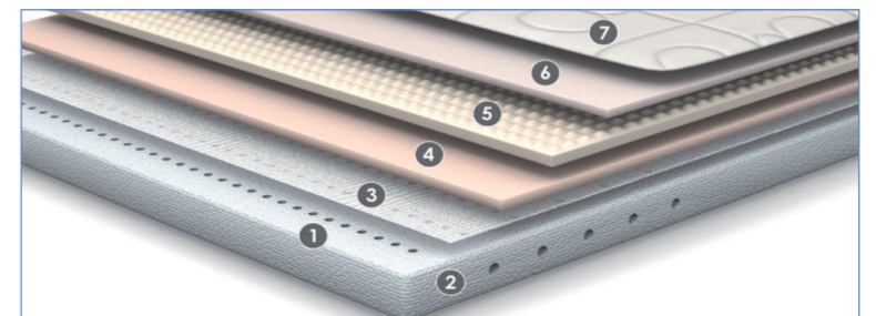
1. Bloque de AirVex® AirPlus 2. Núcleo reforzado 3. Textil NT 4. Poliéter reciclable 5. Sistema Commodo® 6. Fibras hipoalérgicas 7. Tapicería Stretch con tecnología Optigrade® Mismas capas en ambos lados del colchón.
