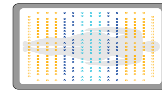
1. Bloque de AirVex® AirPlus 2. Núcleo reforzado 3. Textil NT 4. Poliéter reciclable 5. Sistema Commodo® 6. Fibras hipoalérgicas 7. Tapicería Stretch con tecnología Optigrade® Mismas capas en ambos lados del colchón.
