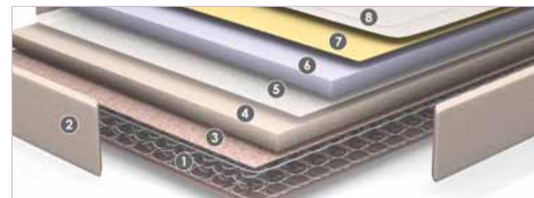
1. Muelle Continuo Multielástico® NxT 2. Encapsulado 3. Filtro 4. Confort System+® 5. Textil NT 6. Sistema Commodo+® 7. Látex 8. Tapicería Strech con tecnología Optigrade®
